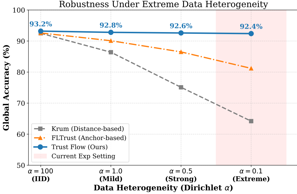
图 10: 环境数据异构度 (Dirichlet \alpha ) 衰减下的各类安全聚合算法鲁棒性压力测试对比
